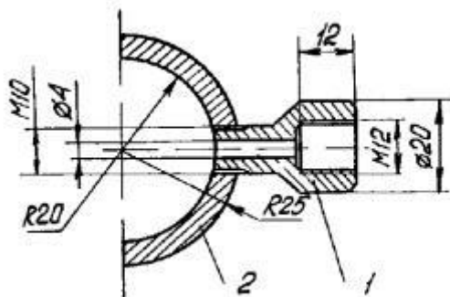
1 - винт; 2 - сектор
